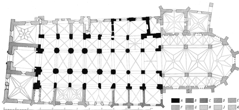
Strängnäs domkyrka, plan med byggnadsperioder. Ur SvK 100.
