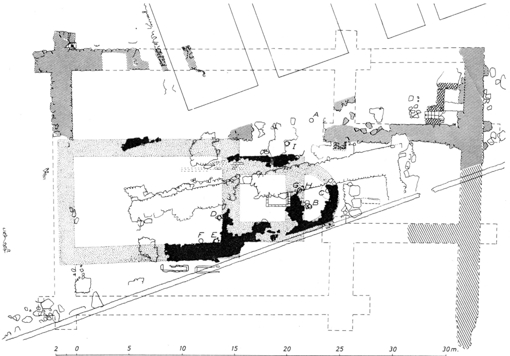
Plansch III. Rekonstruktion av den romanska absidkyrkan och den senmedeltida klosterkyrkans planer. Romanska kyrkan: svart murverk = existerande grundmursfragment; prickade murar = antaglig utsträckning. Klosterkyrkans murar: tät streckning = existerande murar; gles streckning = murar undanröjda vid 1912 års gatuarbeten; krysstreckning = sekundär källare till sakristia?
